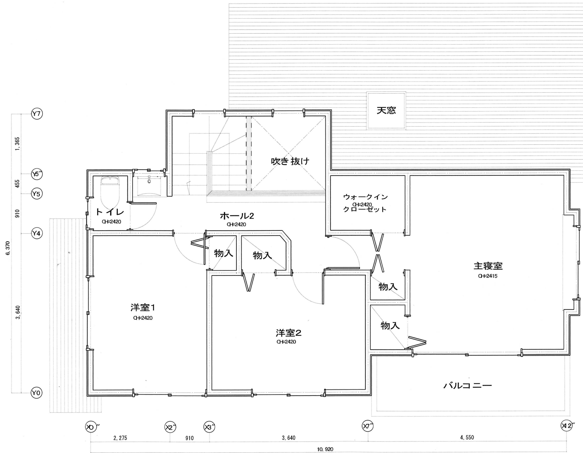
2 階平面図
